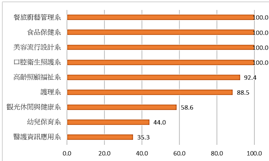
圖 4 最小投入觀點下各 DMU 之 CCR 模式效率值
