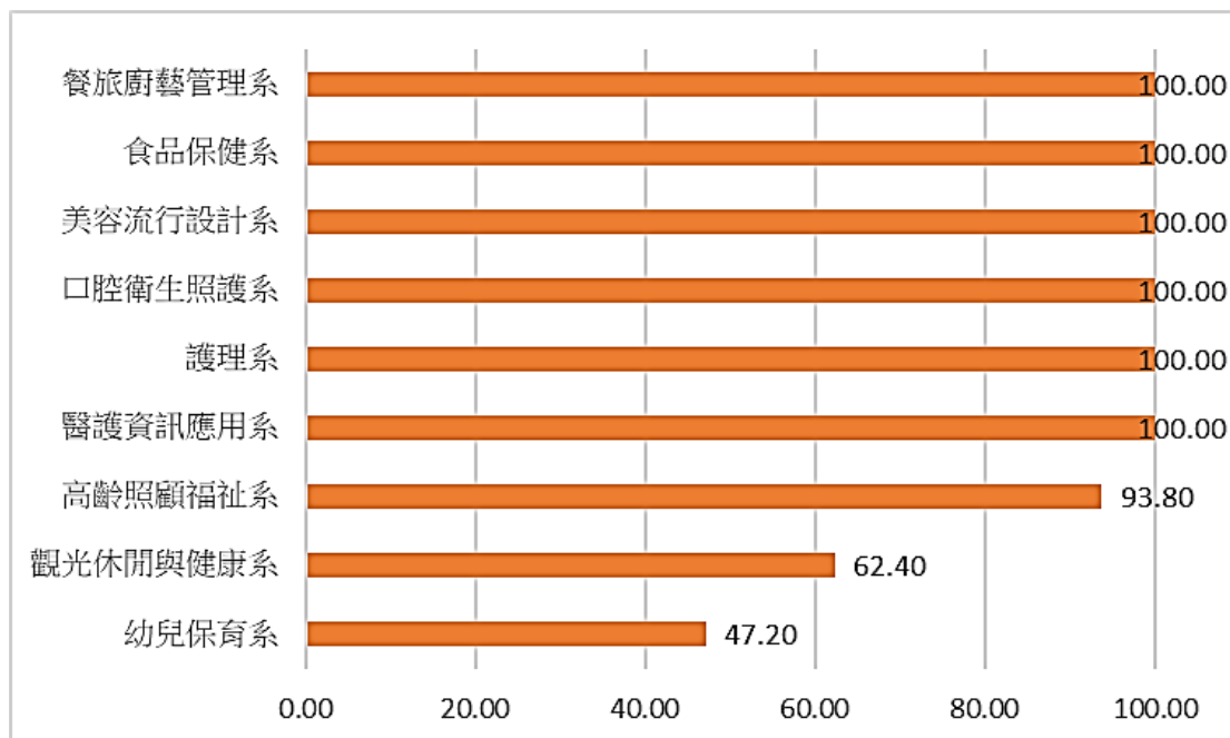
圖 5 最小投入觀點下各 DMU 之 BCC 模式效率值
